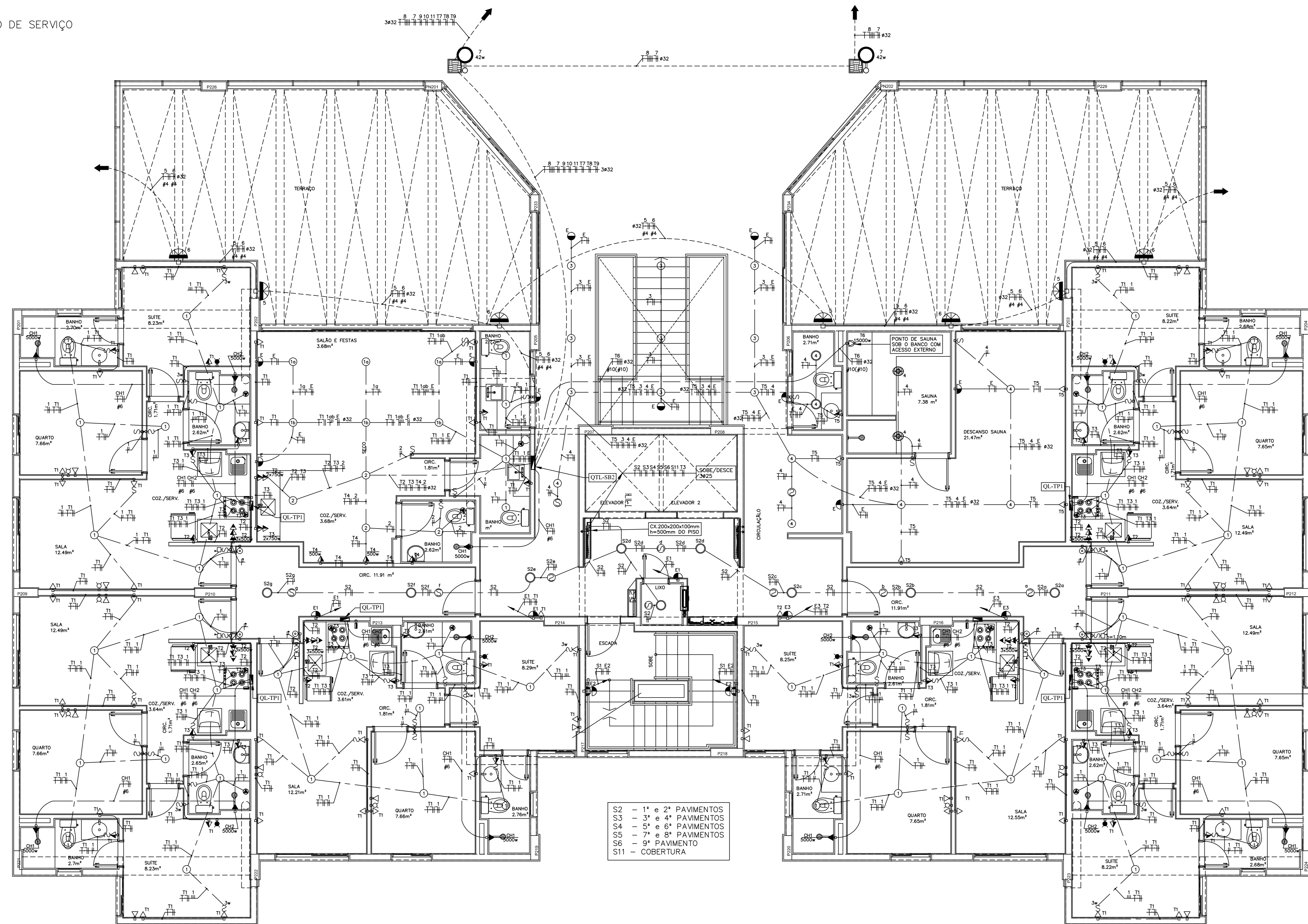
PLANTA BAIXA 1º PAVIMENTO BLOCO B ESCALA 1:50
